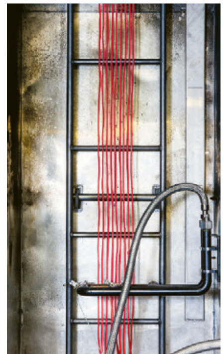
EN 50399 Cable Test Interior detail
